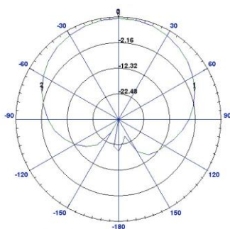
水平面方向圖 H
